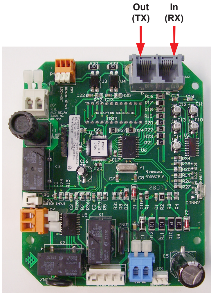
New 3200NT Circuit Board (Not Actual Size)
